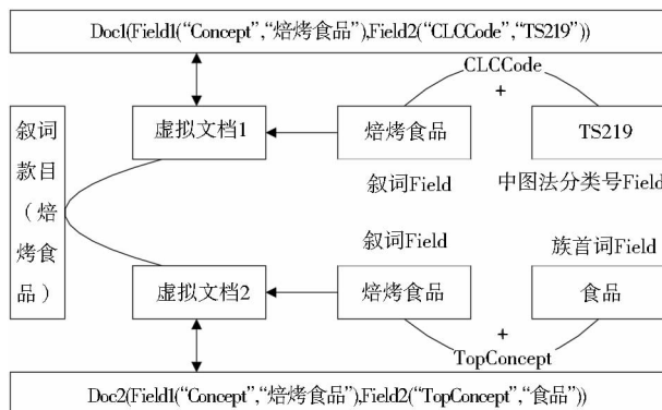
图 3 Lucene 虚拟文档表示的叙词款目信息
