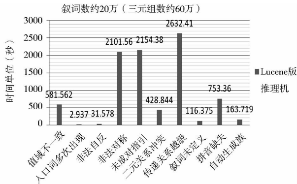
图 10 Lucene 版推理机的效果图
