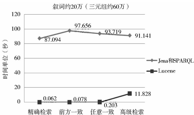
图 8 Lucene 方案与原 Jena/SPARQL 方案的检索效果对比
