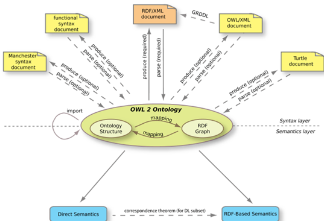
图 1. OWL2 的结构
